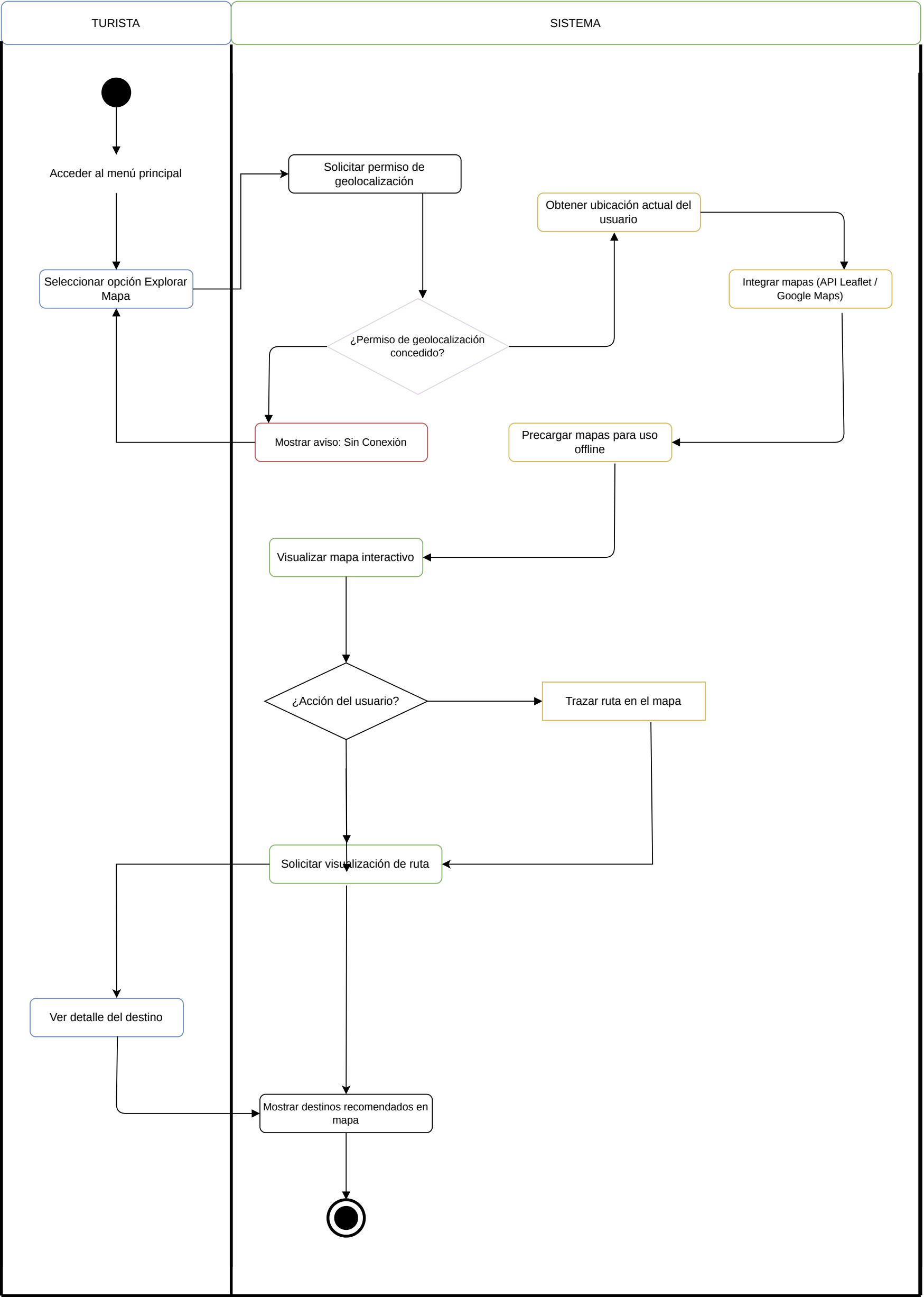
Diagrama de Actividades - RF04: Mapas, Geolocalización y Exploración Espacial
